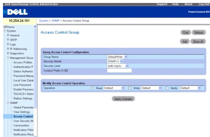
Figure 6-62. Page Access Control Group (Groupe de contrôle d'accès)
